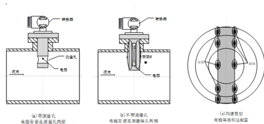
图 1 插入式电磁流量计的结构形式示意图
