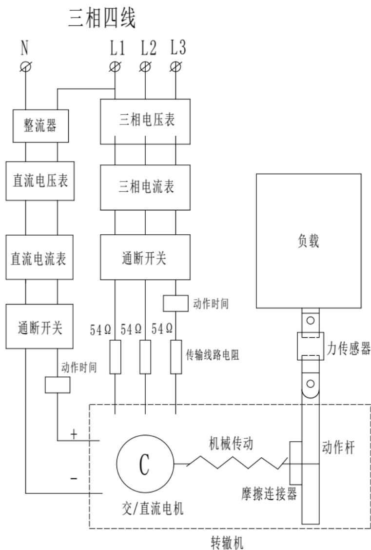
图1 转辙机测试台示意图
