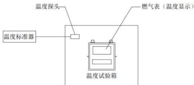
图 2 温度传感器检定示意图
