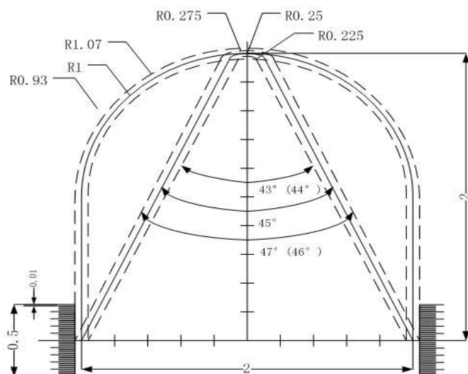
图 2 标准比对样板图
