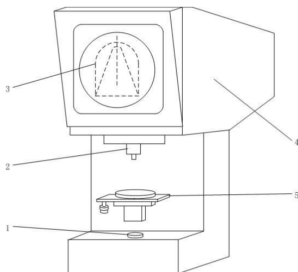
1—光源；2—物镜；3—投影屏；4—外壳；5—移动工作台
