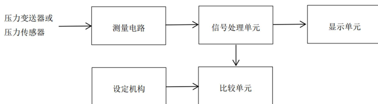
图 1 显示仪的原理框图
