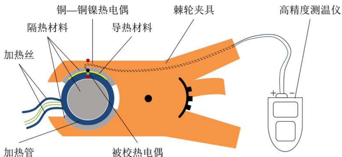
图 E1 加热管型热电偶布置俯视示意图
